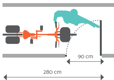
Passage de porte en accès latéral
