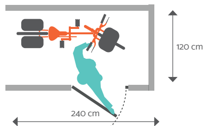
Rangement en accès latéral, en poussant
